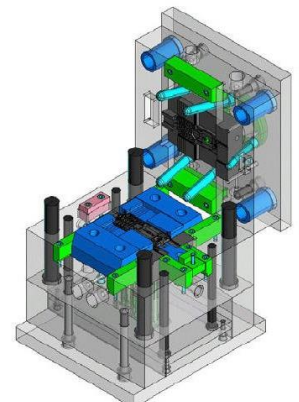
Matrijsconstructie als 3D file
