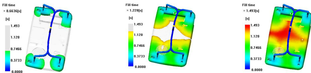
Füllanalyse; Hilfsmittel zur Bestimmung der Position der Anspritzpunkte
